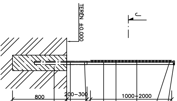
ŘEZ J-J
